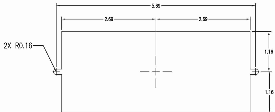
UTS1 CUTOUT TEMPLATE
